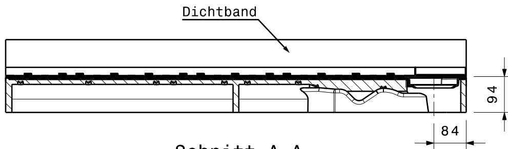
Schnitt A-A
