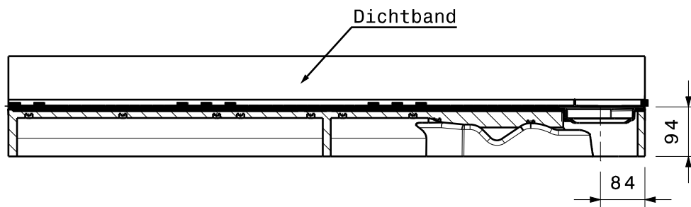
Schnitt A-A
