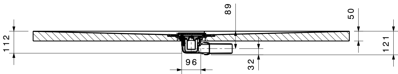
Schnittansicht A-A
