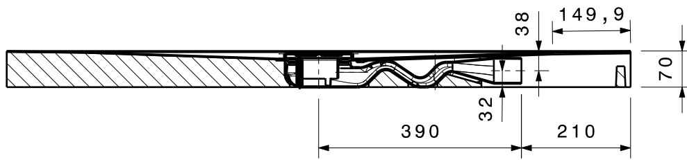
Schnitt A-A
