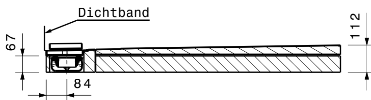
Schnitt B-B
