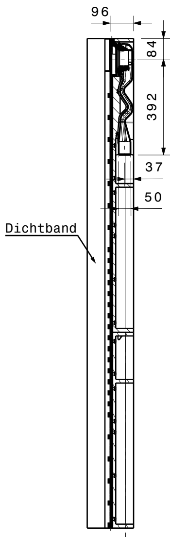
Schnitt A-A
