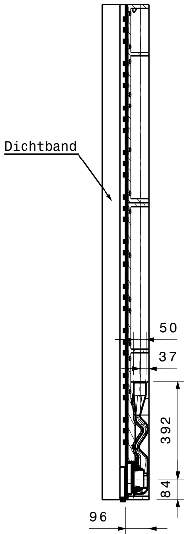
Schnitt B-B
