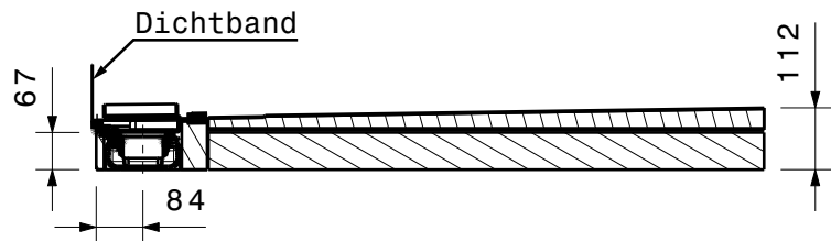
Schnitt A-A
