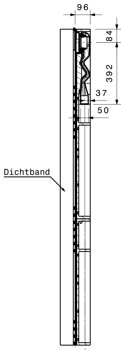
Schnitt B-B
