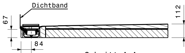
Schnitt A-A
