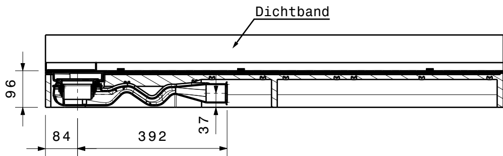
Schnitt A-A
