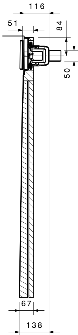
Schnitt B-B
