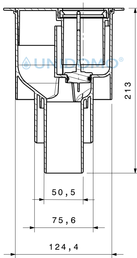
Schnitt A-A
