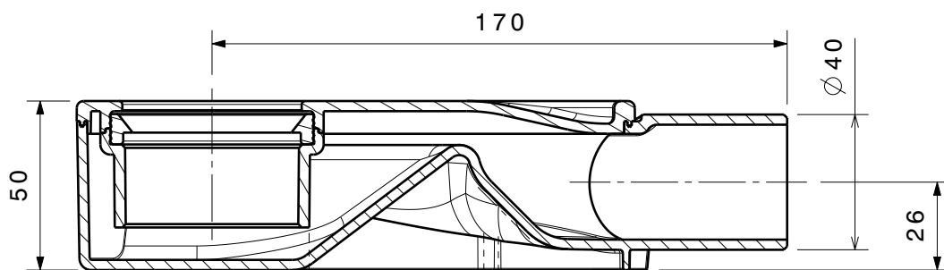
Schnitt A-A
