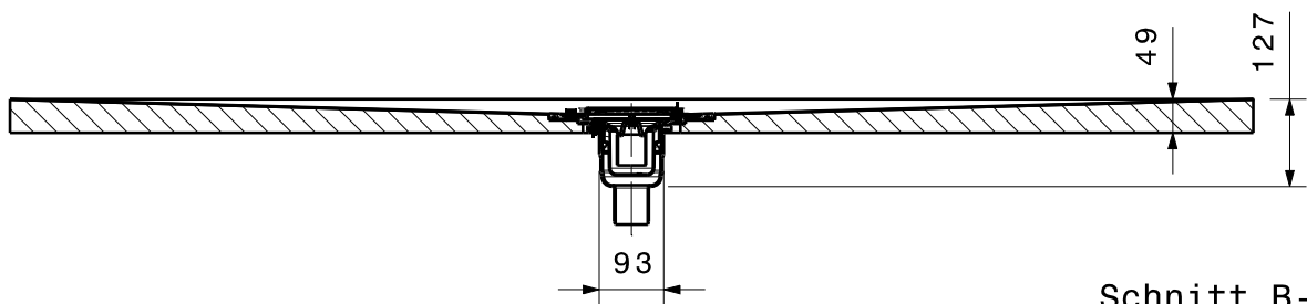
Schnitt B-B
