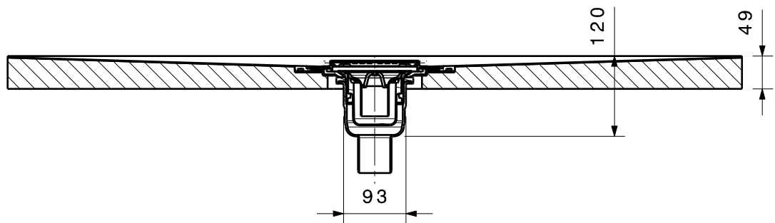
Schnitt B-B
