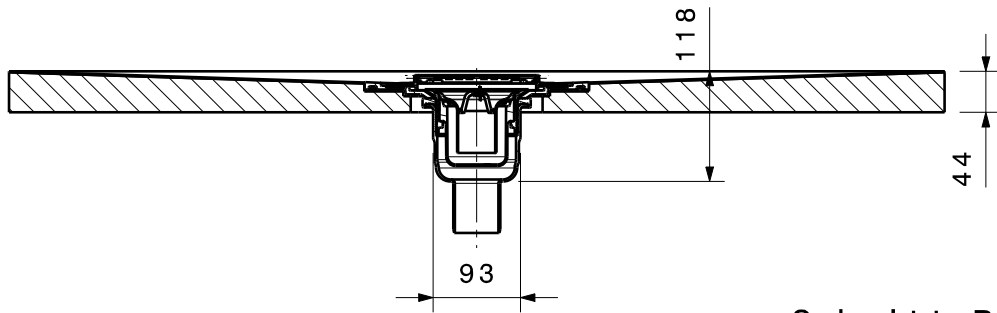
Schnitt B-B
