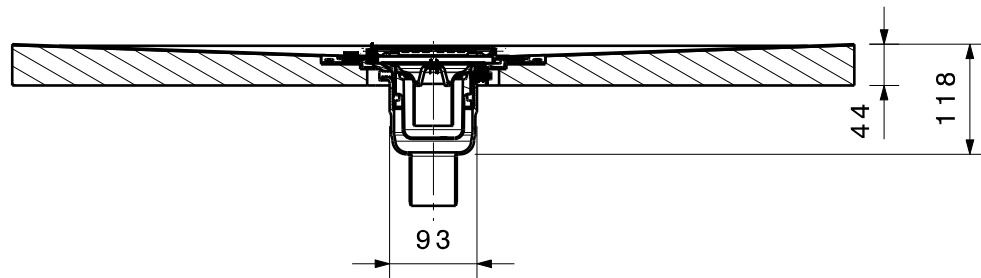
Schnitt B-B
