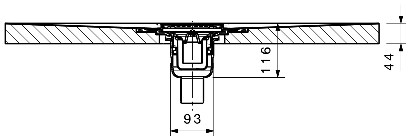
Schnitt B-B
