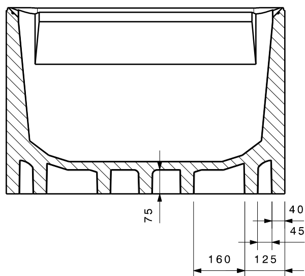
Schnittansicht A-A[2]
