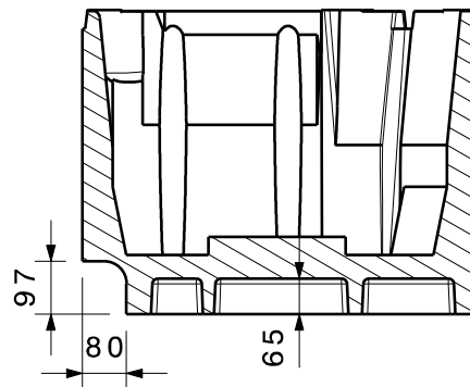
Schnittansicht A-A
