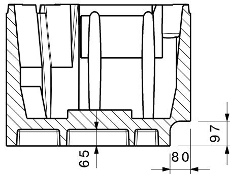
Schnittansicht A-A
