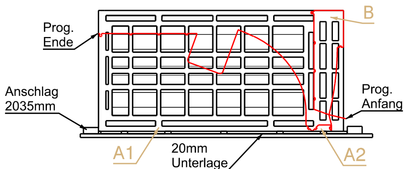
Position Konturenschneider
