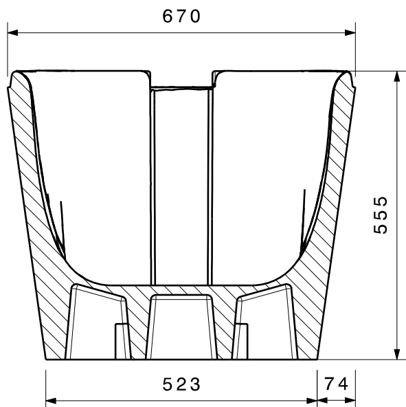
Schnittansicht A-A[2]
