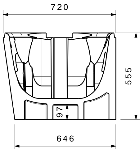
Schnittansicht A-A
