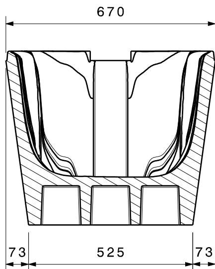
Schnittansicht A-A
