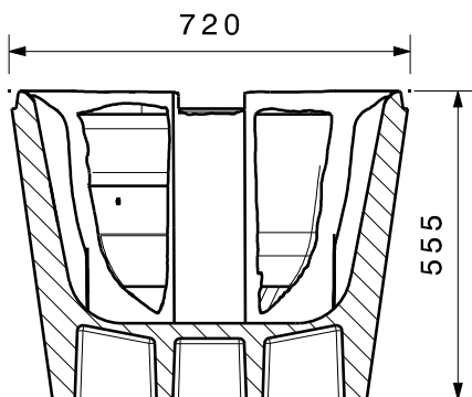
Schnittansicht A-A[2]
