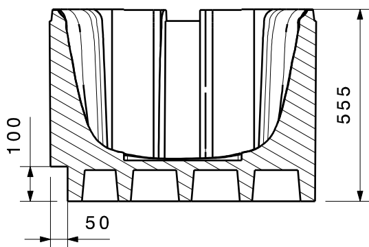
Schnittansicht A-A[2]
