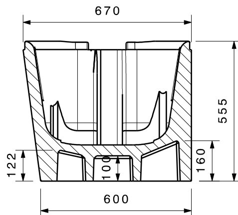
Schnittansicht A-A
