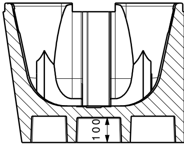
Schnittansicht A-A
