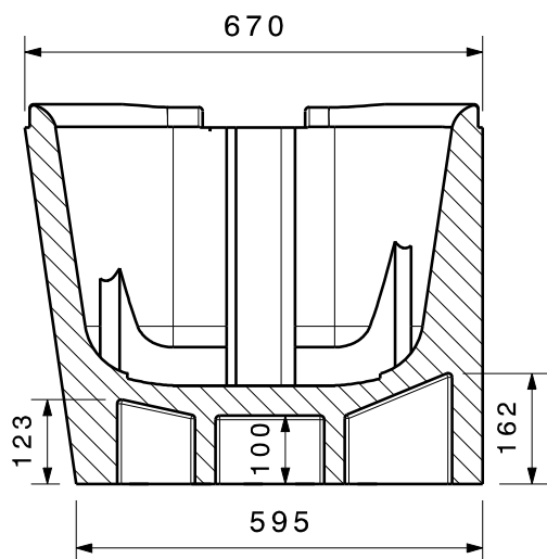
Schnittansicht A-A
