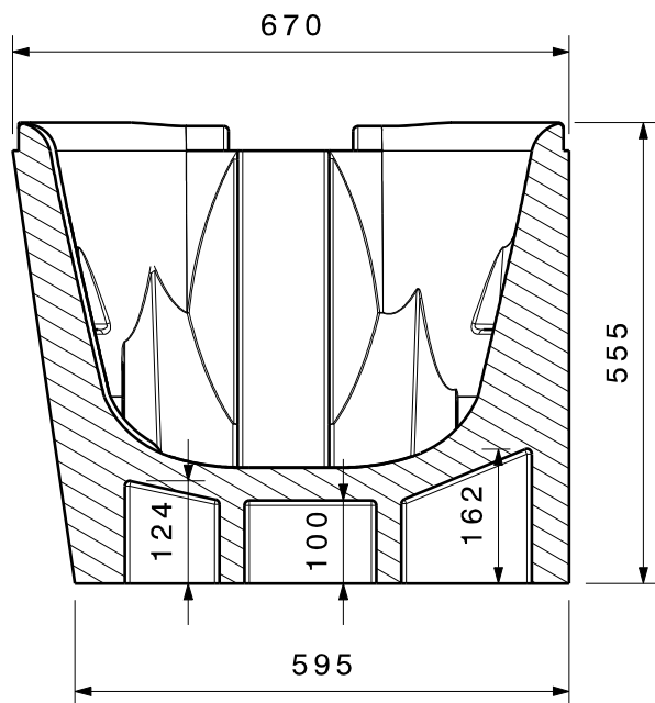
Schnittansicht A-A
