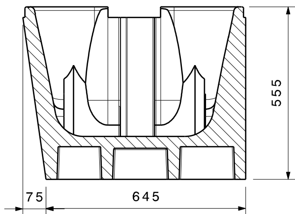
Schnittansicht A-A[2]
