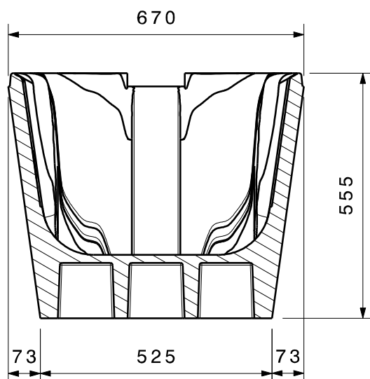
Schnittansicht A-A[2]
