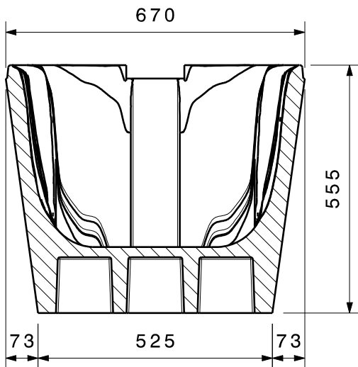
Schnittansicht A-A[2]
