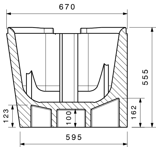
Schnittansicht A-A
