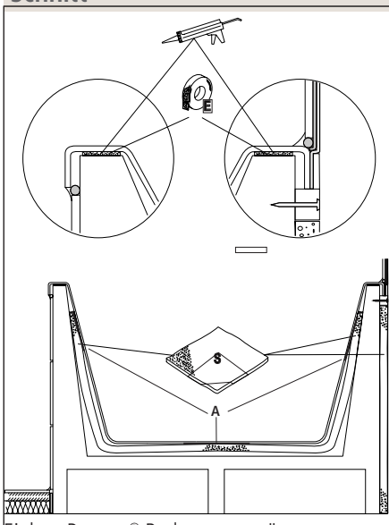
Einbau Poresta® Badewannenträger
