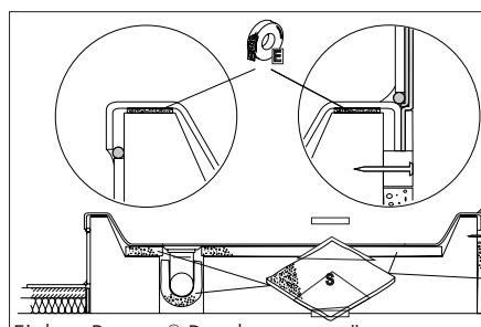
Einbau Poresta® Duschwannenträger
