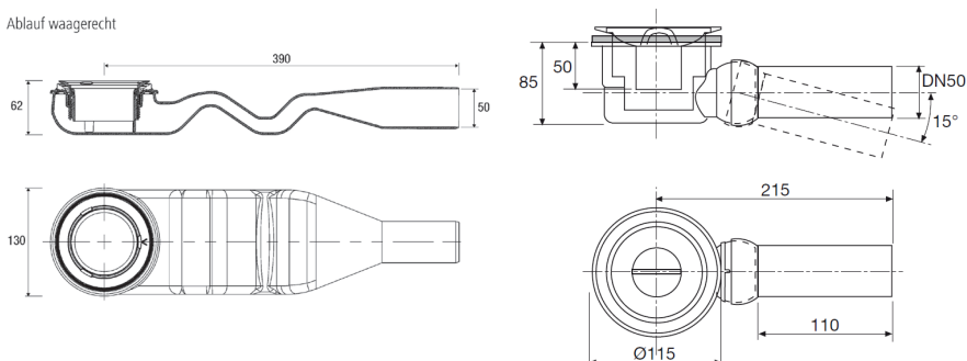
Ablauf waagrecht
