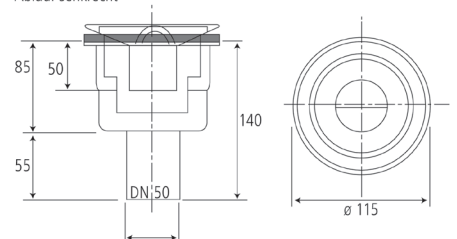
Ablauf senkrecht
