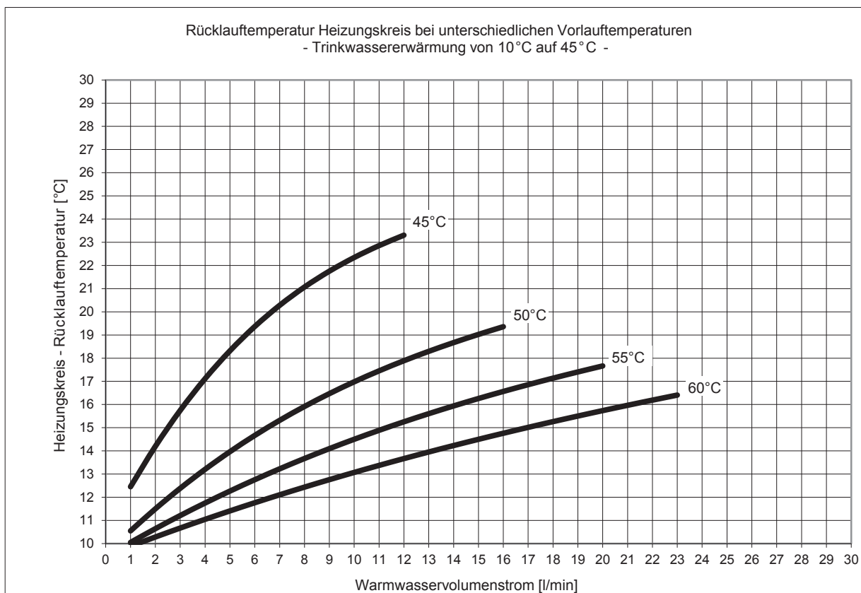
Abb. 11: Leistungsbereich 1, Trinkwassererwärmung auf 45 °C (Leistungsangaben gem. SPF-Prüfprozedur)
