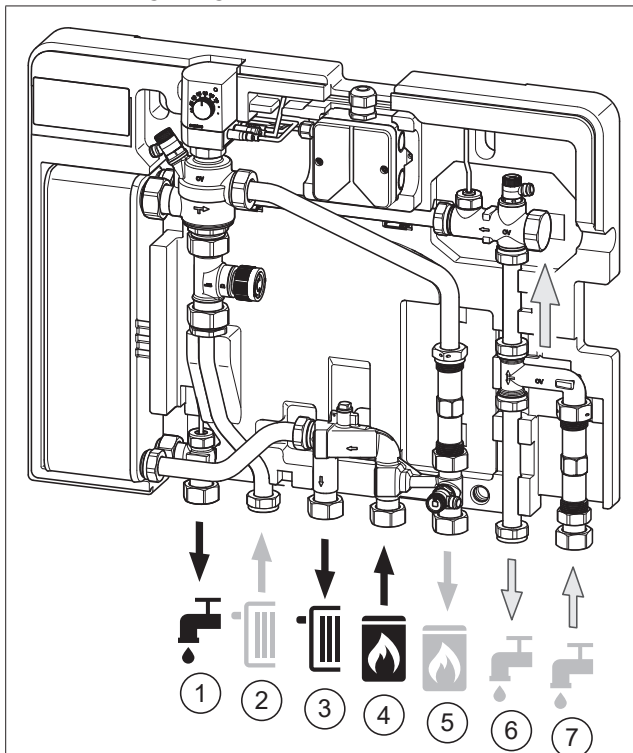
Abb. 1: Anschlussbelegung
