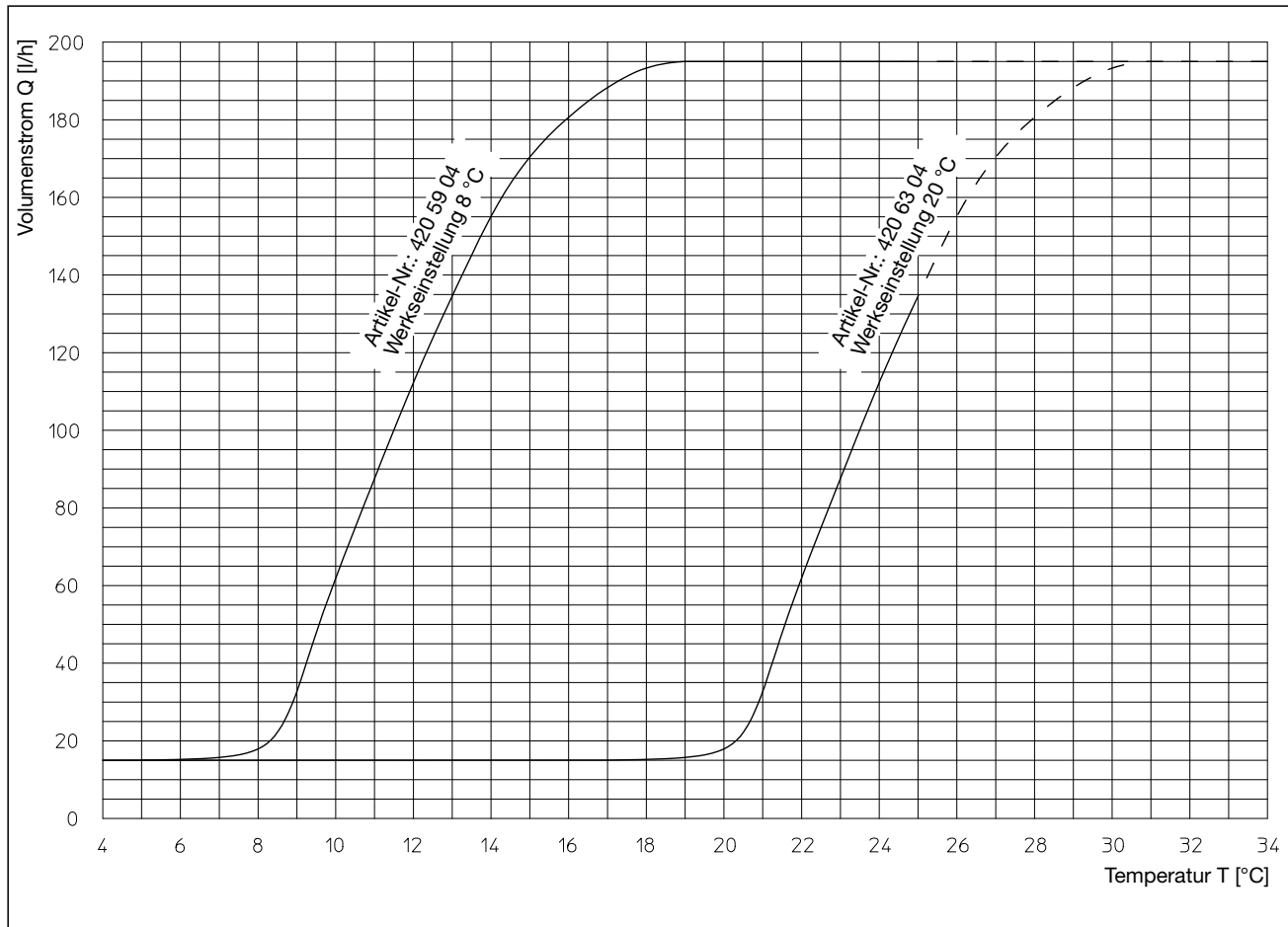
Regelcharakteristik „Aquaström K“ (gemessen bei \Delta P = 100 \text{ mbar} )
