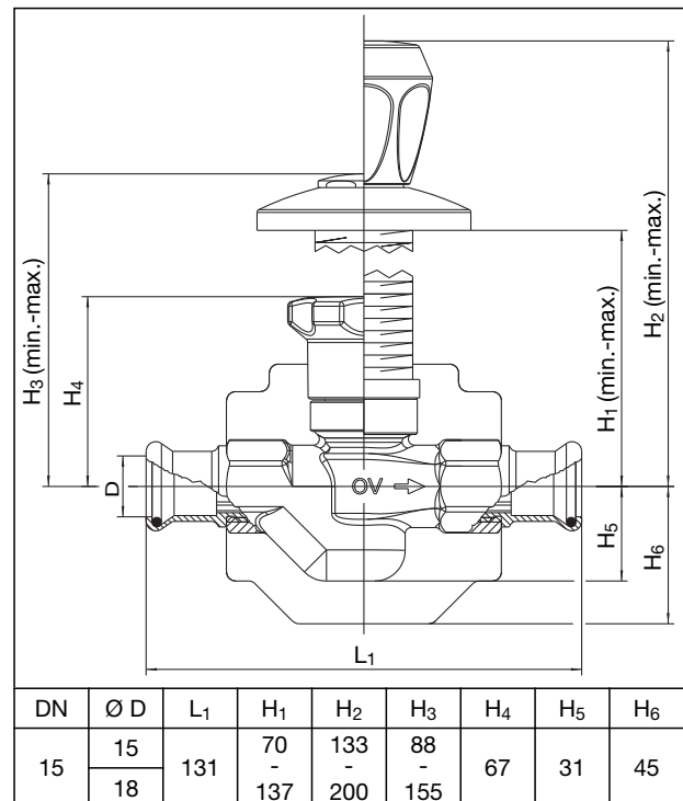
Maße „Aquastrom UP-Therm“ mit Pressanschluss
