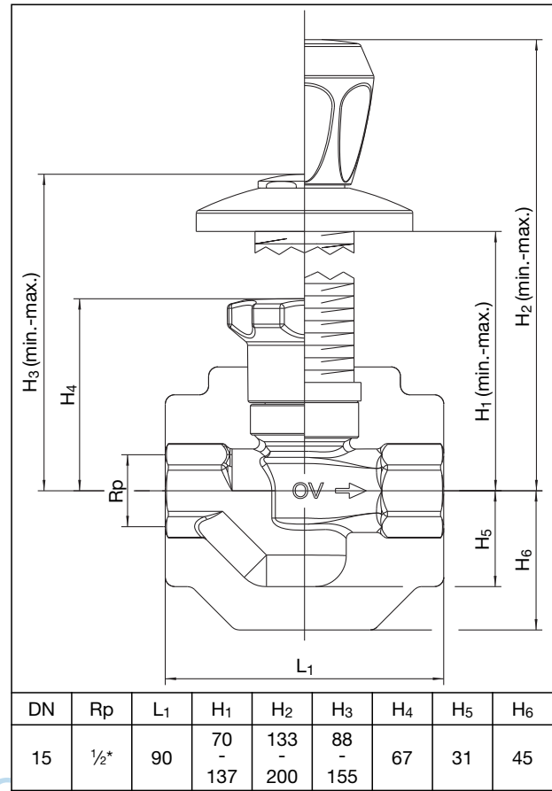
Maße „Aquastrom UP-Therm“ Innengewinde
