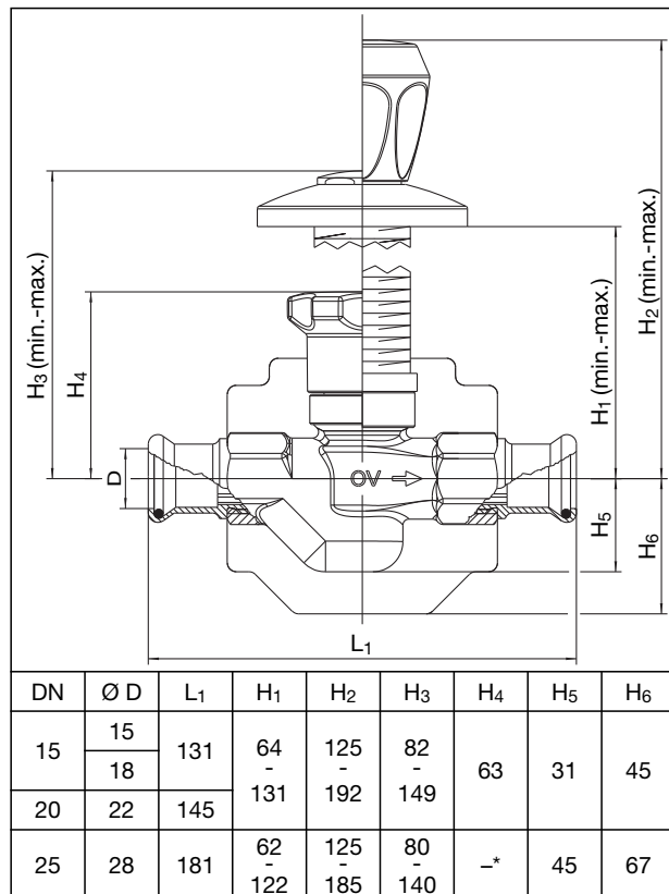
Maße „Aquastrom UP-F“ mit Pressanschluss
