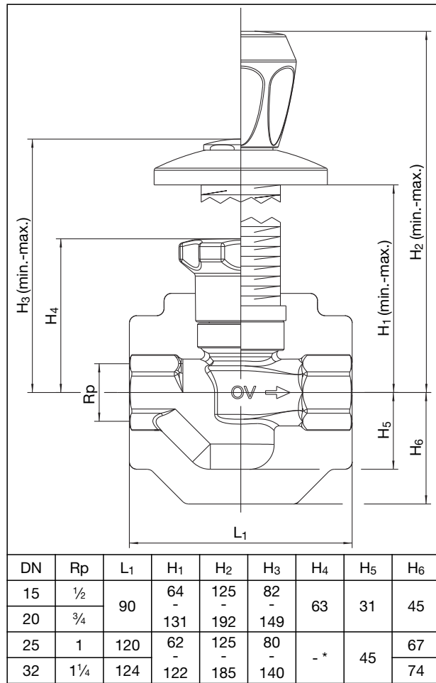
Maße „Aquastrom UP-F“ Innengewinde
