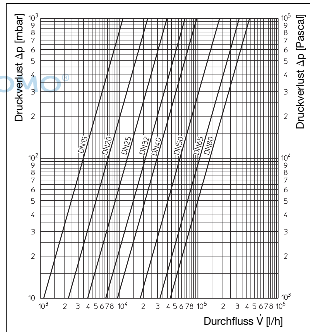
Durchflussdiagramm
