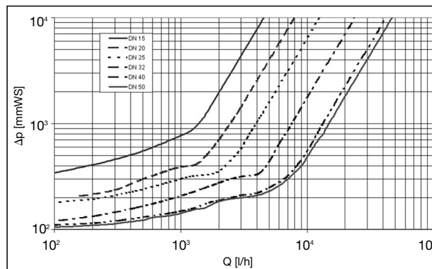
Druckverlustdiagramm
