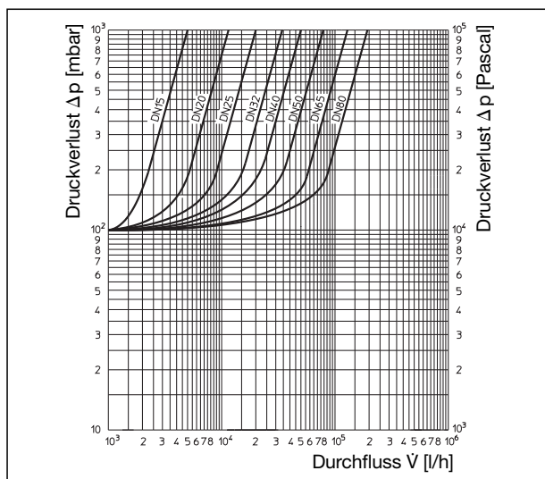
Durchflussdiagramm „Aquaström KFR“
