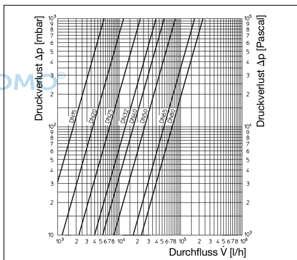
Durchflussdiagramm „Aquaström F“
