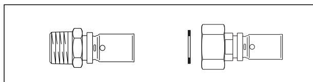
„Cofit P“ Verbindungstechnik für Innen- und Außengewindeanschluss
