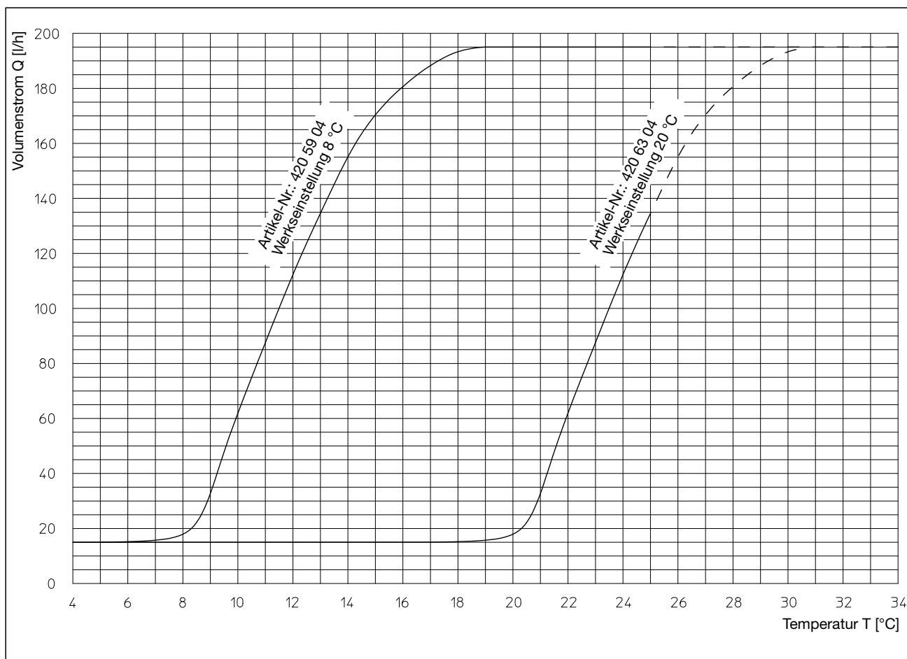
Regelcharakteristik „Aquaström K“ (gemessen bei \Delta P = 100 \text{ mbar} )
