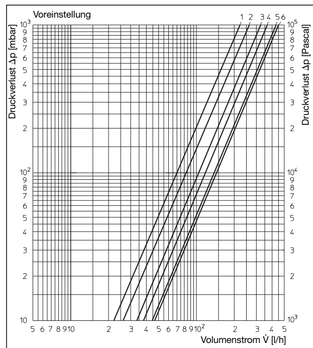
„Aquaström VT“ DN 20 Desinfektionsvolumenstrom
