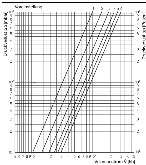
„Aquaström VT“ DN 20 Restvolumenstrom
