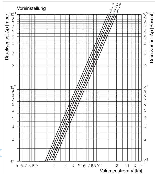
„Aquaström VT“ DN 15 Desinfektionsvolumenstrom
