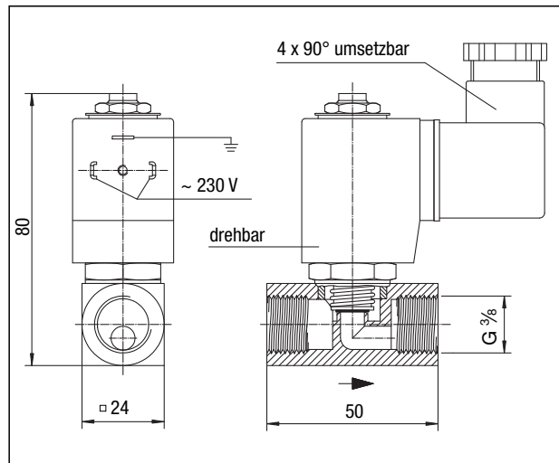
Maße „Oilstop MV“
