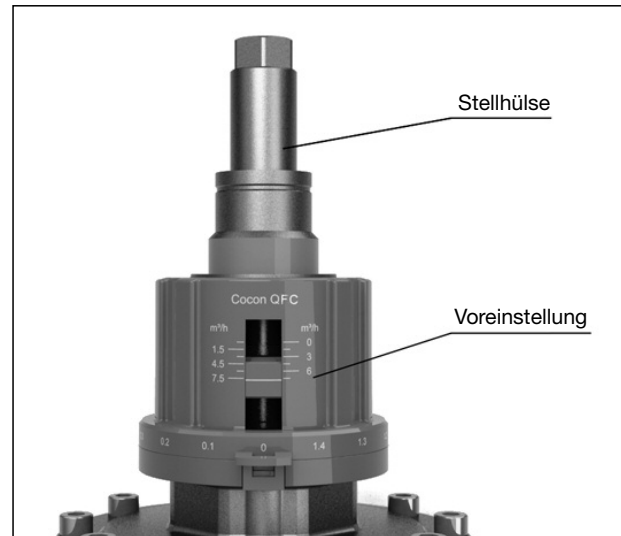
Stellhülse
