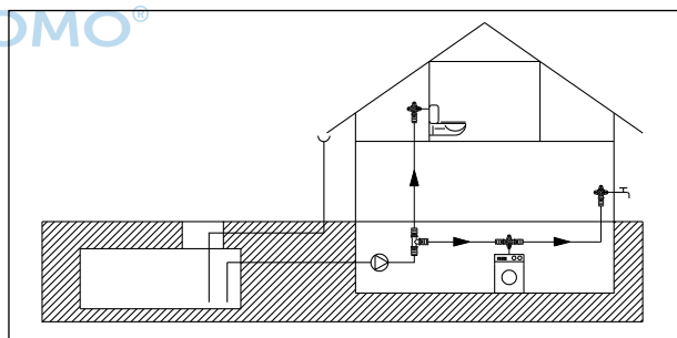
System-Darstellung Regenwassernutzung
