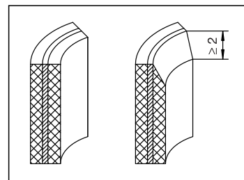
Vor dem Entgraten: links nach dem Entgraten: rechts
