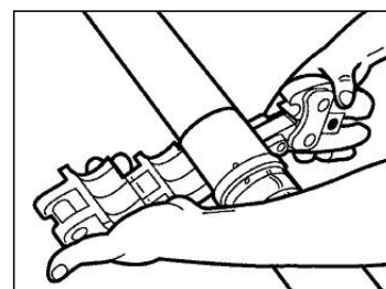
Presskette um Presshülse legen (63 mm)
