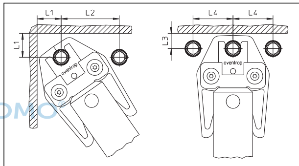
Oventrop Press-Werkzeuge
