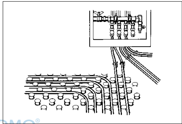
System-/Noppenplatte
