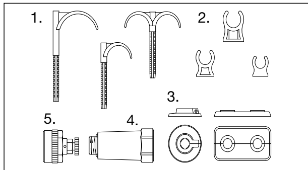
Oventrop Verlegematerial
