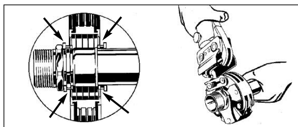
Press-Werkzeug ansetzen
