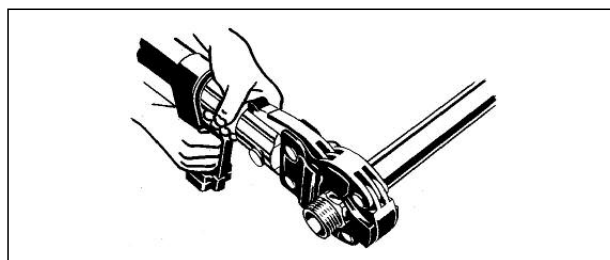
Verpressung durchführen
