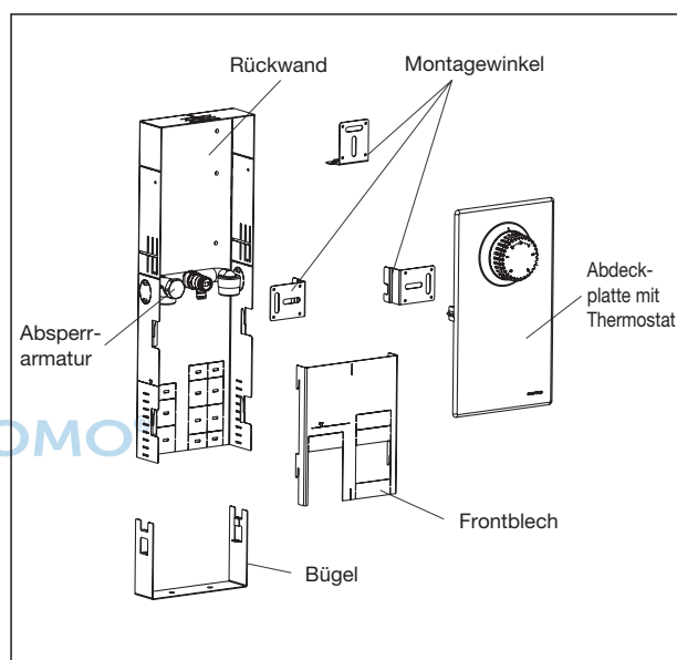
Übersicht Montagekanal
