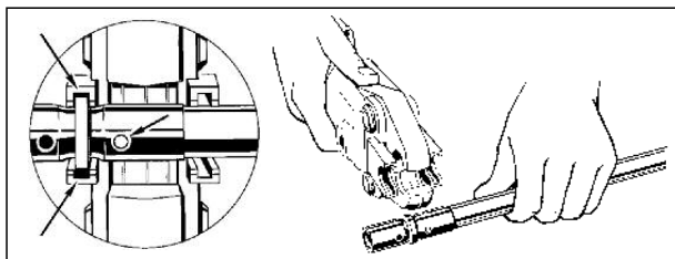
Press-Werkzeug ansetzen
