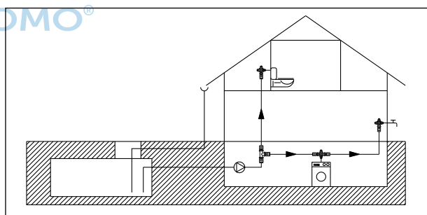
System-Darstellung Regenwassernutzung
